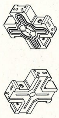
Détail C 10:1
